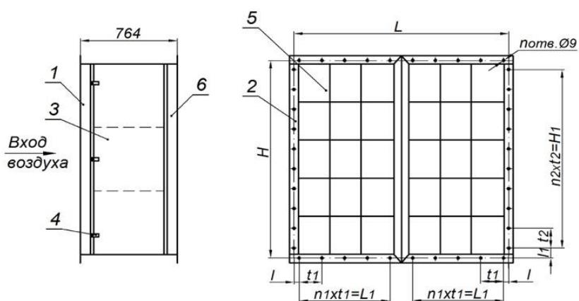
Рис.3 Схема секции карманного фильтра СКФ 2/6х5; 2/6х6
